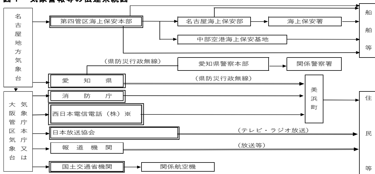
図1 気象警報等の伝達系統図
