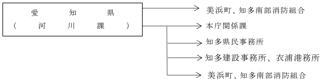
図3 水位周知海岸の水位情報（高潮氾濫発生情報）
