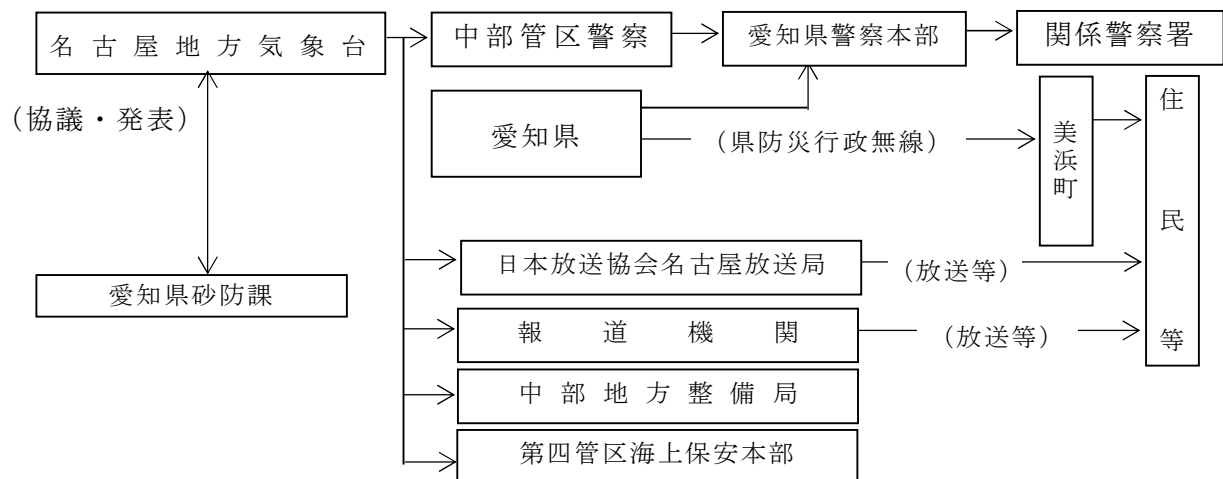
図4 土砂災害警戒情報（警戒レベル4相当情報〔土砂災害〕）
