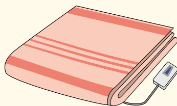
電気毛布
