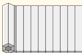
風呂ふた
