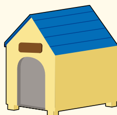
犬小屋
