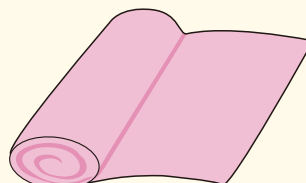
カーペット
