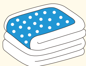
ふとん
