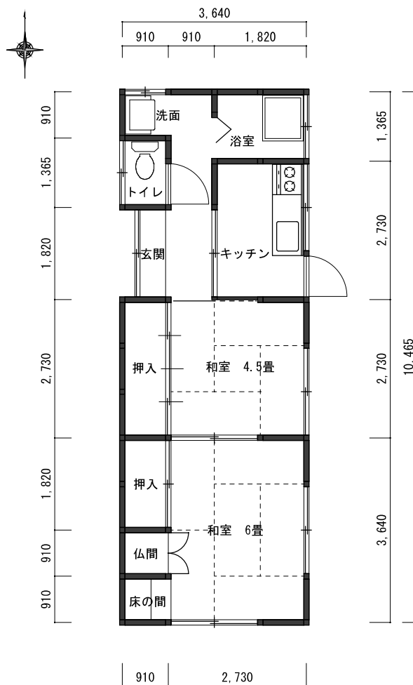
平面図 S=1/100
